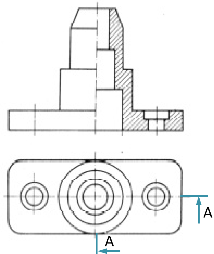
Presjek A-A
