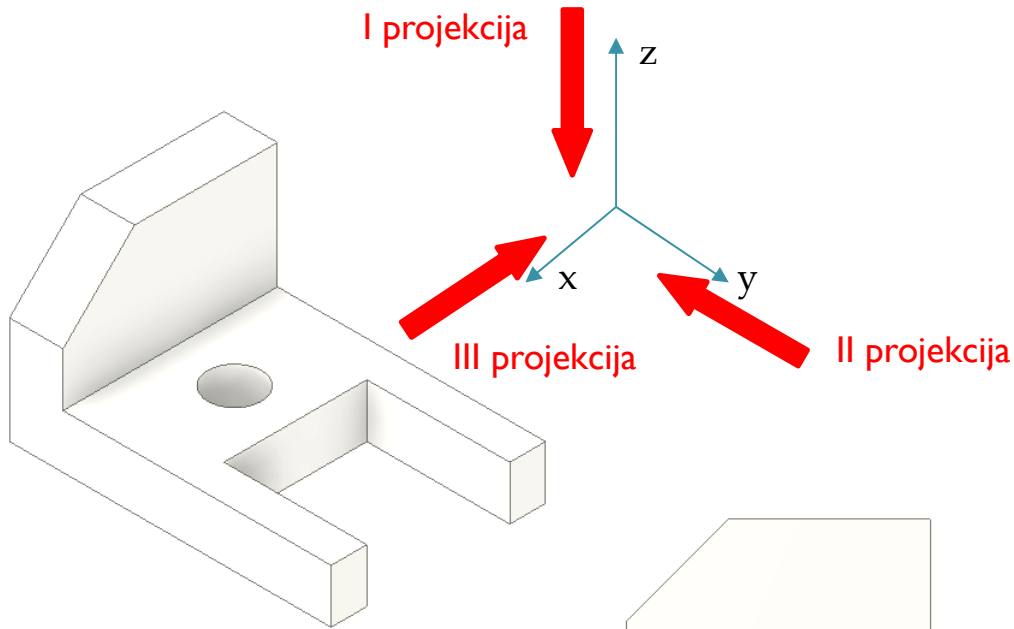
II projekcija
